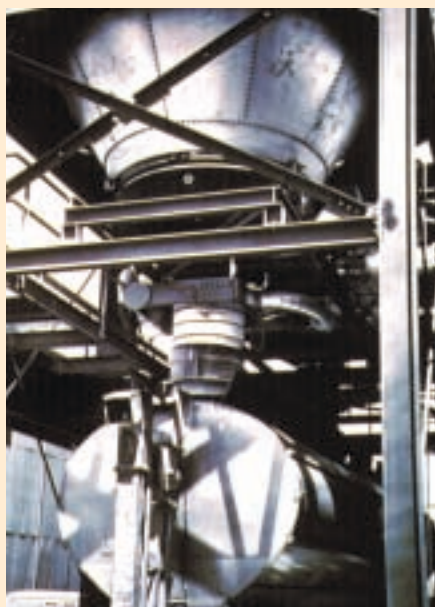
▲ハッチ付タンクローリー車積みの例
